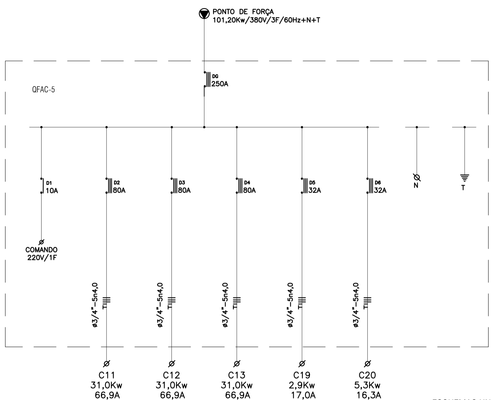
ESQUEMAS UNIFILARES QFACS
